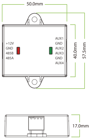
Aux485/WR485
